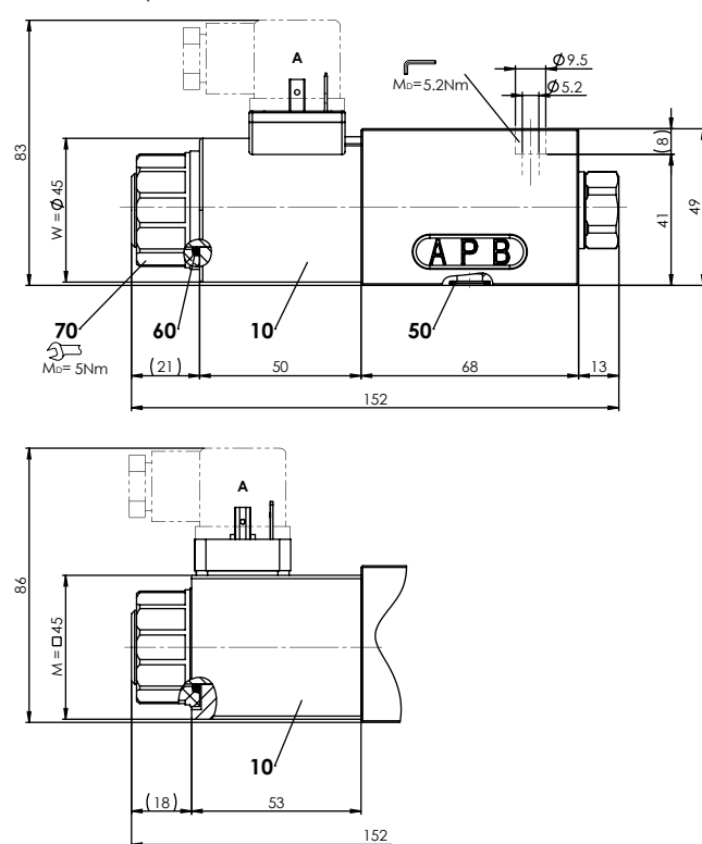
Distributeur 4/2-voies
